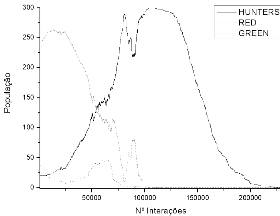
Figura 39. Extinção devido ao consumo total dos recursos.
